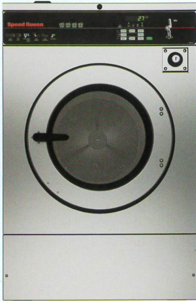
SC-E40 洗濯機 20kg
